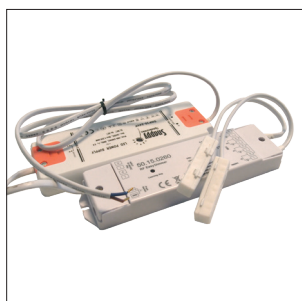
Transfo. + E/R radio LED2 > min 1 spot / max 12
